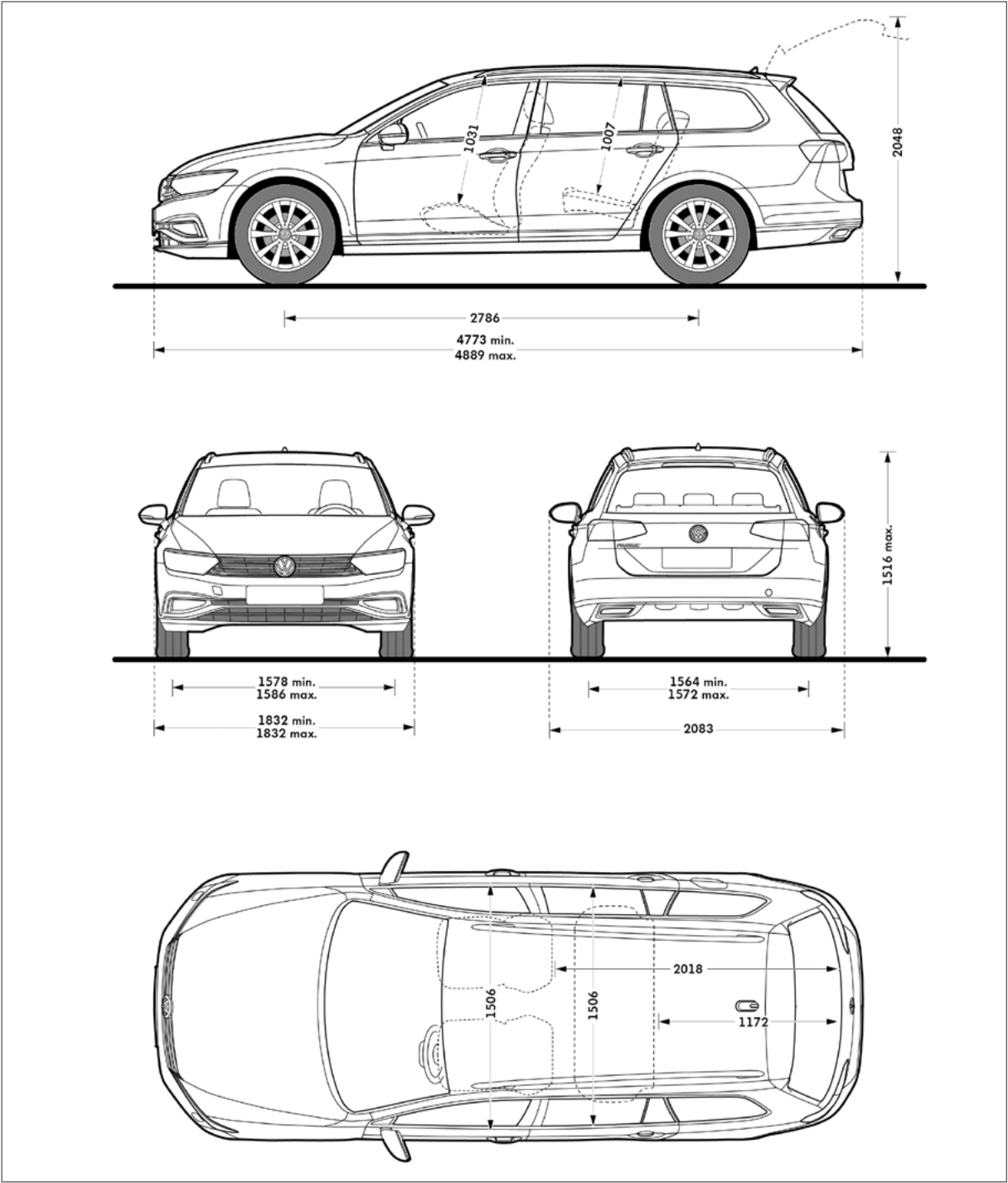
Sur les illustrations, lorsque les flèches et les chiffres sont montrés à l'intérieur du véhicule, les mesures sont pour les dimensions intérieures. Lorsque les flèches et les chiffres sont montrés à l'extérieur du véhicule, les mesures sont pour les dimensions extérieures. Remarque : les illustrations présentées ne reflètent pas nécessairement les spécifications de la France.
